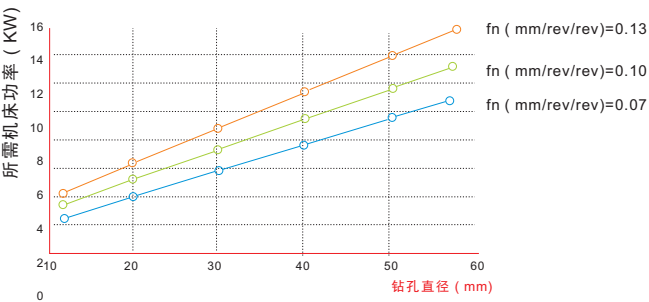
快速钻头切削数据参考表
