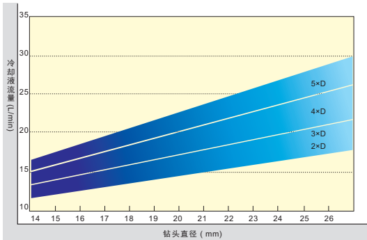
加工功率要求
