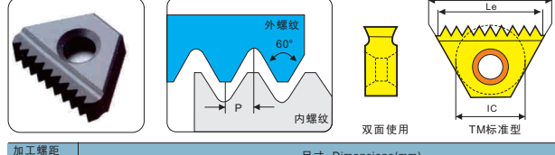
UN-60° 美制统一标准螺纹铣刀片 UN-60°American UN Full Profile
