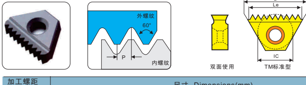
UNJ 美制航空航天机械螺纹铣刀片 UNJ Aviation Thread
