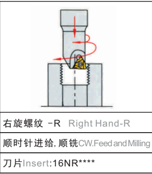
内螺纹铣削方法 Internal thread milling method
