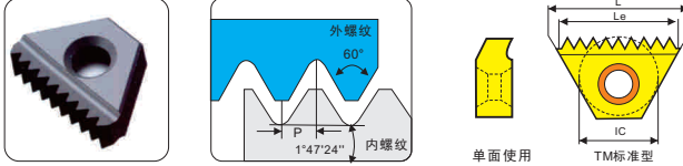
NPT 美国标准锥管螺纹铣刀片 NPT-60°National Pipe Threads
