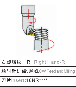
外螺纹铣削方法 External thread milling method
