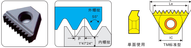
BSPT 英国标准锥管螺纹铣刀片 BSPT-55°
