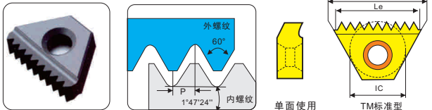
NPTF 美制干密封螺纹铣刀片 NPTF(Dry seal)
